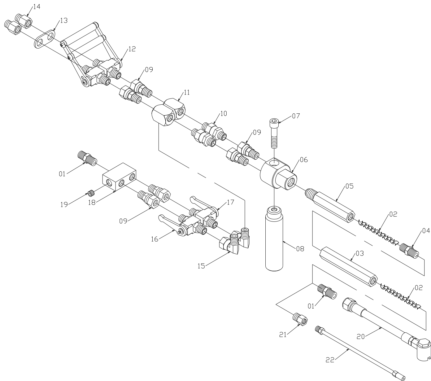
分解圖:3P-LG-01
