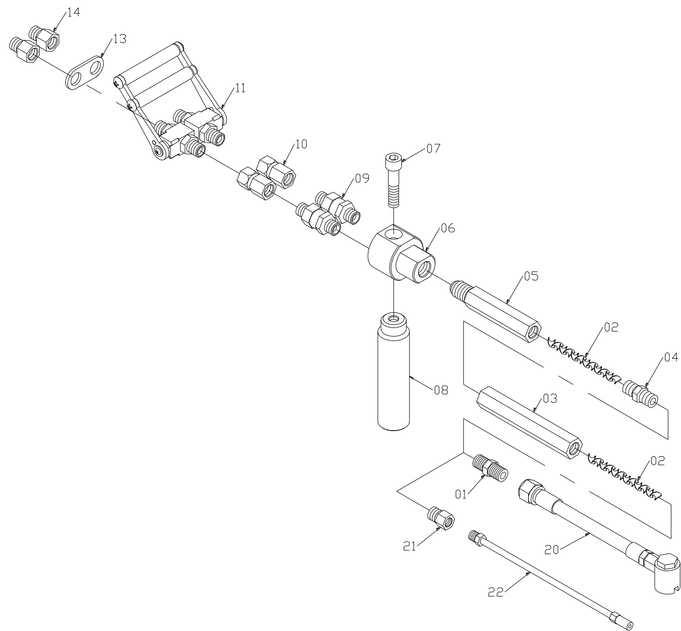
分解圖:2P-LG-01
