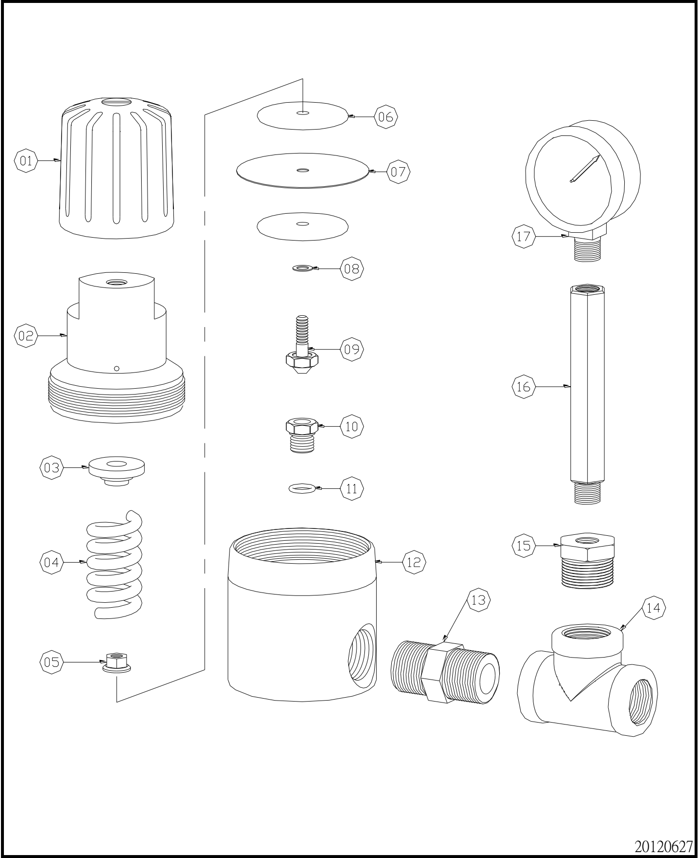
分解圖：
